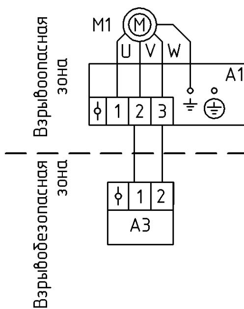
Рис.Б.2 – Схема подключений блока конденсаторов А3 к двигателю (для МЭО ...-0)
